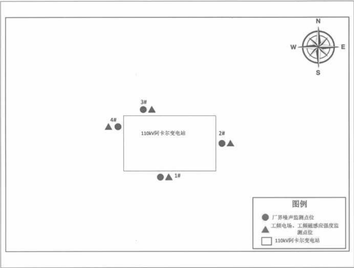
附图 1 2023 年第五师 83 团新建及改造 110 千伏输变电农村电网巩固提升工程验收监测（电磁辐射、噪声）点位示意图
