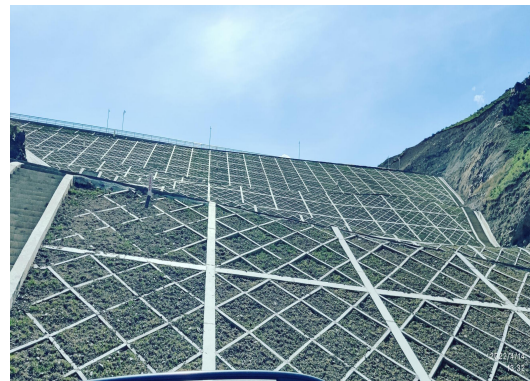
护坡
